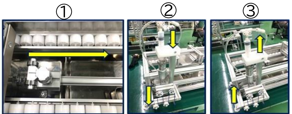
①W/Bが流れると下部にあるスライダーが動く
