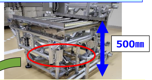
動滑車・定滑車を使用して重量1/4
