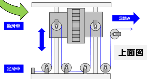
動滑車・定滑車を使用して重量1/4
