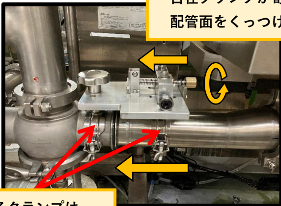
各クランプは 同じ高さの為、 高さ合わせができる
